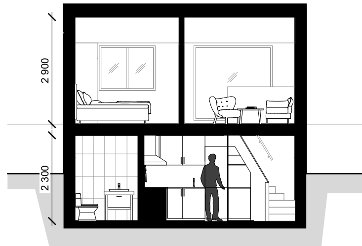
LÄNGDSEKTION
